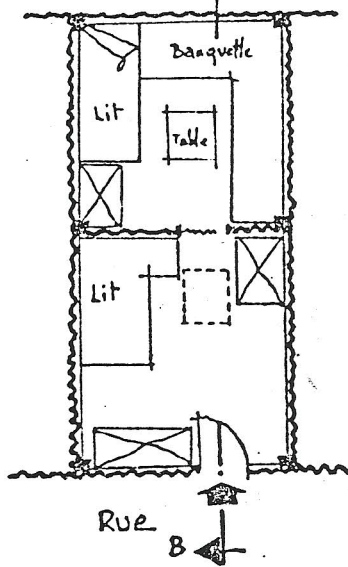
TYPE 2
